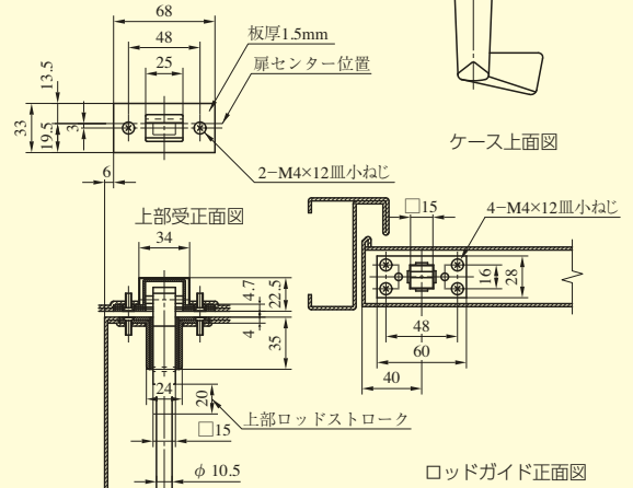
ロッドガイド正面図
